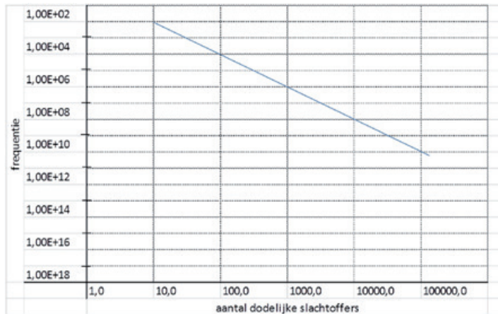
Figuur 7.1 / Veiligheidsnorm zoals vastgelegd in de Warvv.
